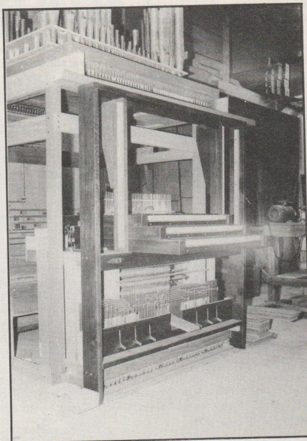
Kijkje in de werkplaats waar het huispijporgel van de heer Bonefaas in opbouw is
